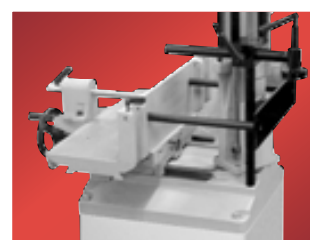
Set comprenant la butée et le dispositif de pression vers le bas pour un travail à 180° (No. d'art. 719 A-MDA)
